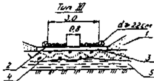
Графическая схема 2. Усиление ледовых переправ деревянным настилом: 1 - снеговой покров; 2 - колесопроемы; 3 - поперечины; 4 - естественный ледяной покров; 5 - вода
